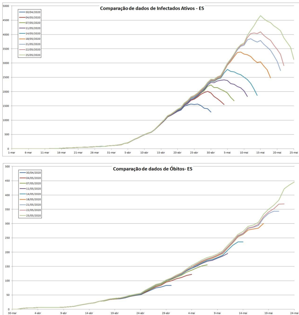
Figura 8 – Comparação de dados de infectados ativos (topo) e óbitos (base) com datas-bases entre 30 de abril e 25 de maio
