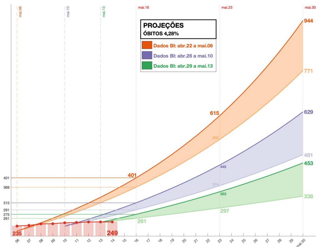
Figura 2 – Projeções de óbitos (dados observados até 14/05)
