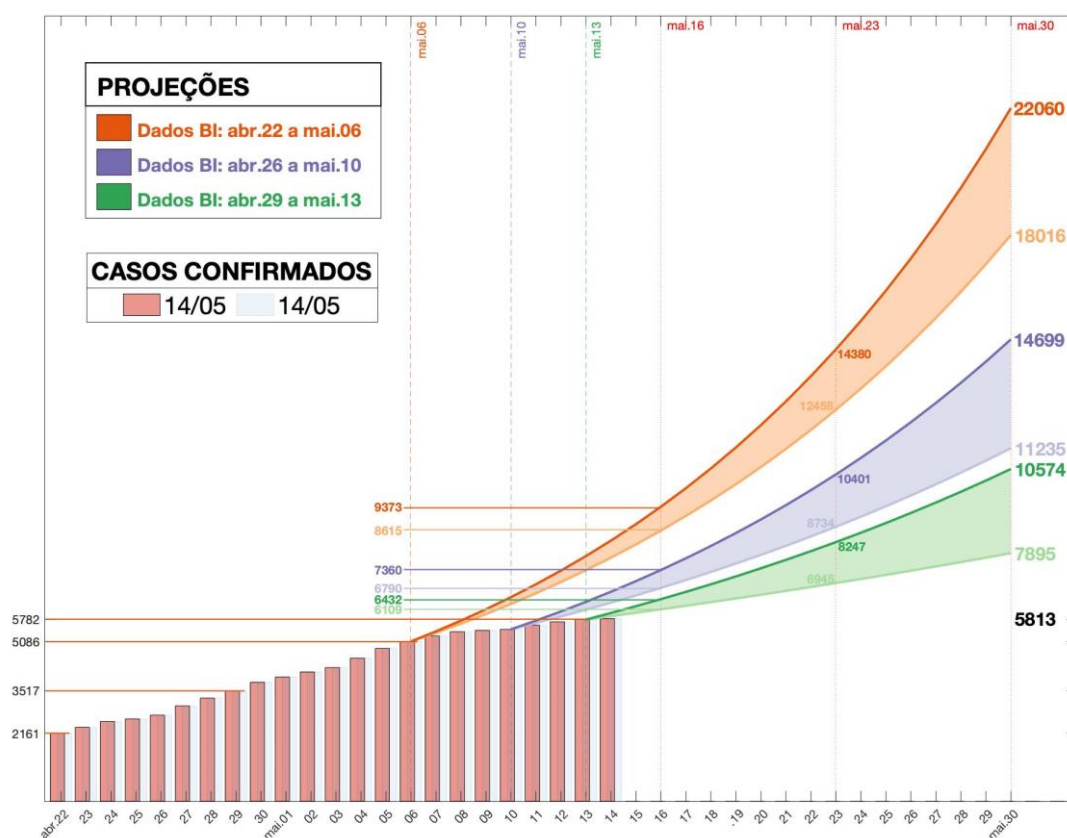
Figura 1 – Projeções de casos confirmados (dados observados até 14/05).
