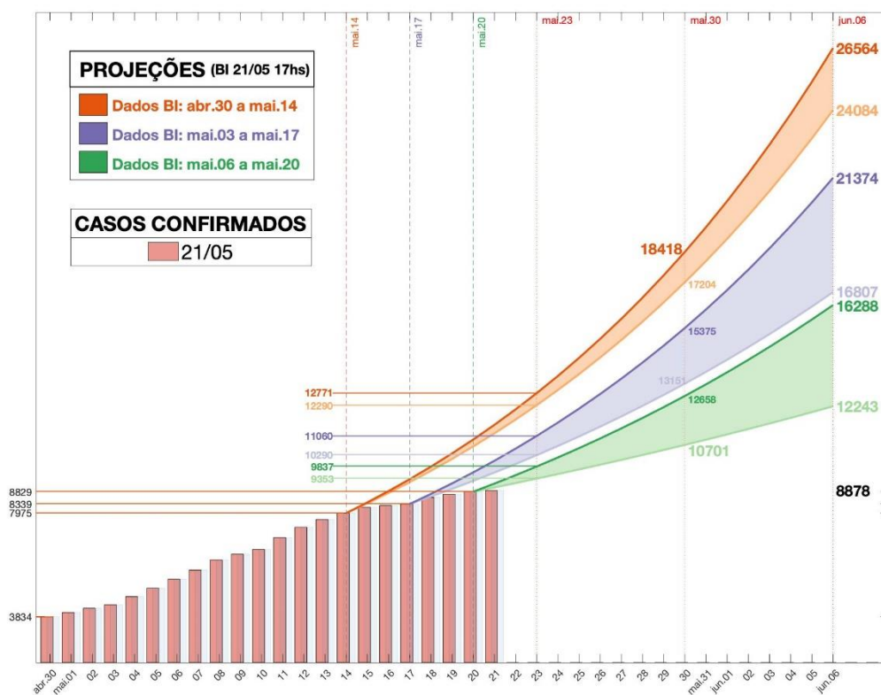
Figura 5 – Projeções de casos confirmados (data-base 21 de maio)
