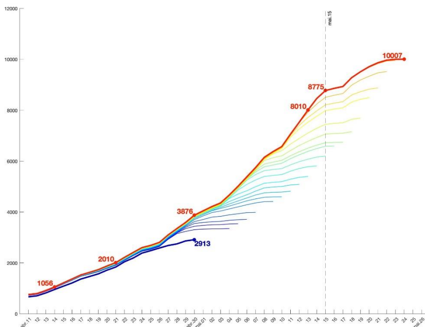
Figura 7 – Evolução dos casos confirmados no Painel COVID-19 com datas-bases entre 30 de abril e 24 de maio
