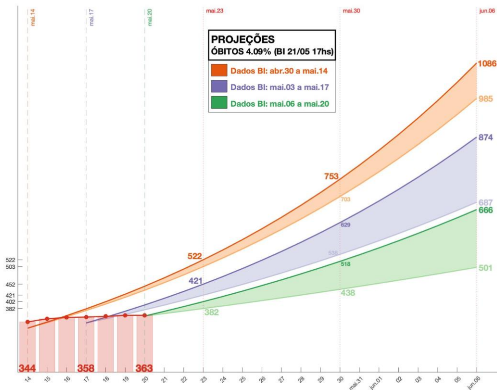
Figura 6 – Projeções de óbitos (data-base 21 de maio)
