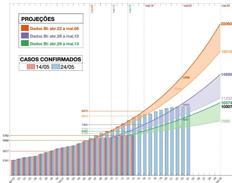
Figura 3 – Projeções de casos confirmados e atualização de dados observados até 24/05
