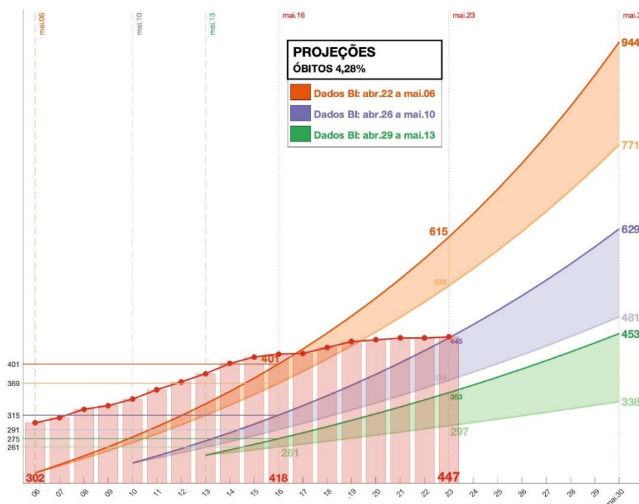
Figura 4 – Projeções de óbitos e atualização de dados observados até 24/05
